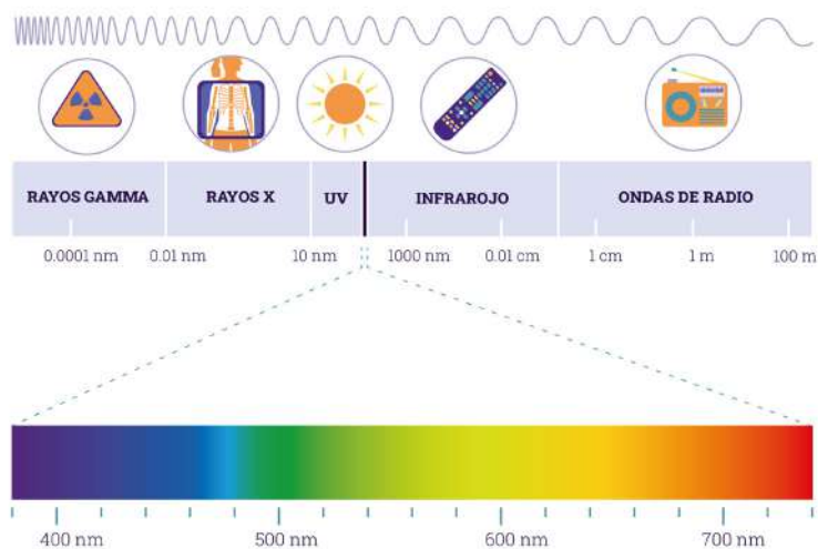
Gráfico 2 Espectro electromagnético destacando la franja del visible
